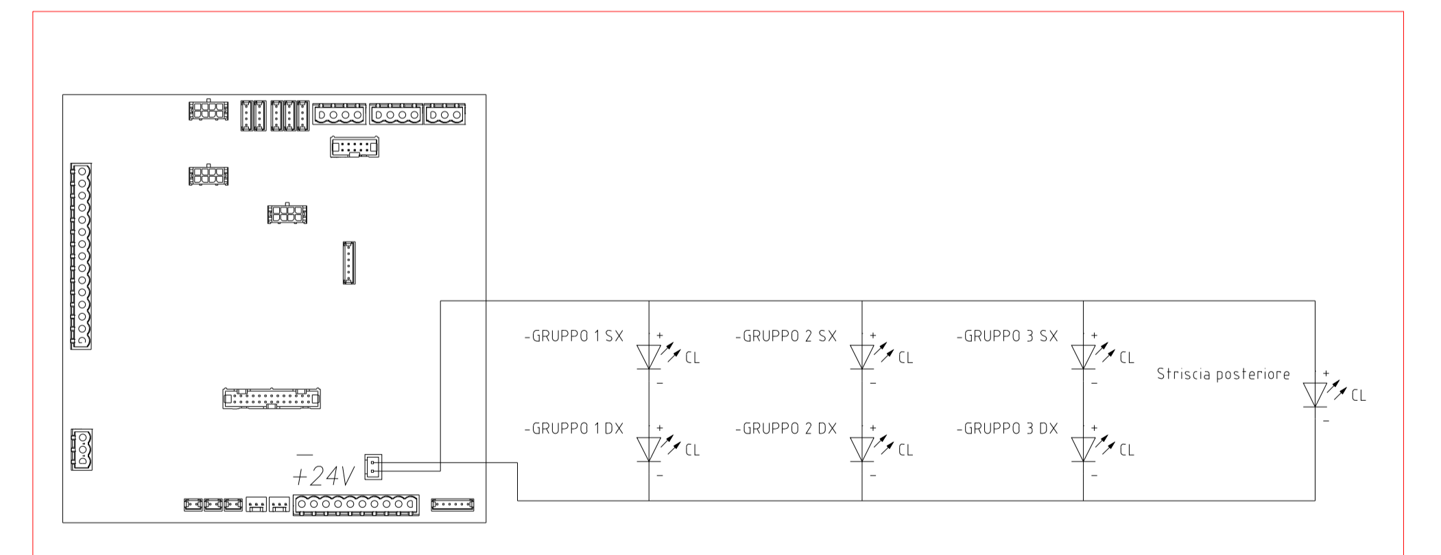
SCHEMA ELETTRICO "LUCI EAGLE ONE" 2-3 GRUPPI
